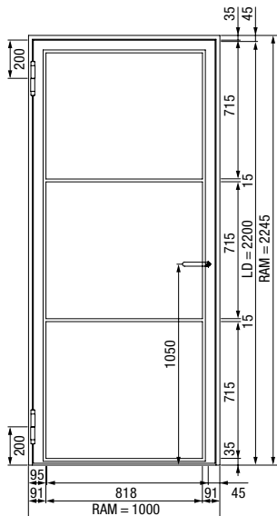
1-krídlové oceľové dvere Loft
