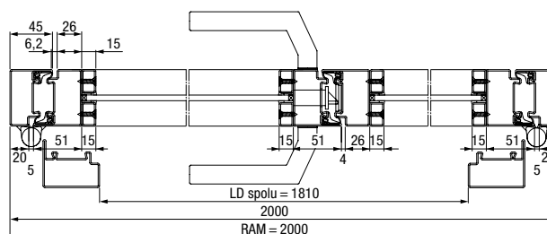
Horizontálny rez 2-krídlové oceľové dvere Loft
