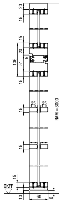
Vertikálny rez 1-krídlové oceľové dvere Loft s bočnými dielmi a nadsvetlíkom
