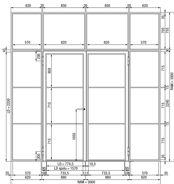
2-křídlové ocelové dvěre Loft s bočnými dielmi a nadsvetlíkom
