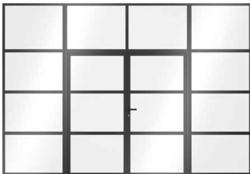
2-krídlové s bočnými dielmi a nadsvetlíkmi, uhlová zasklievacia lišta
